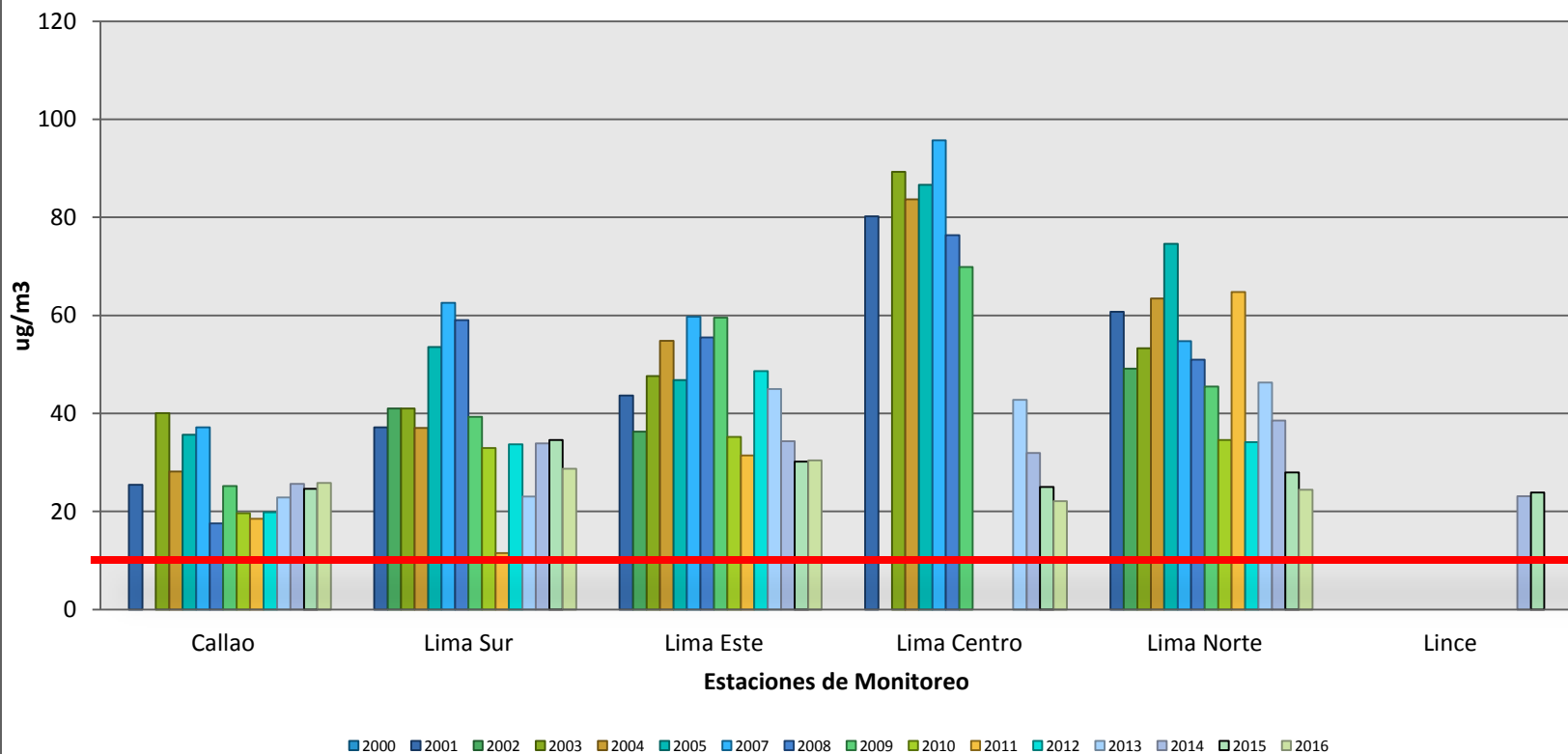
Comportamiento Anual de PM2.5 en las estaciones de la Red de Vigilancia en Lima - Callao Años 2000 - 2016
