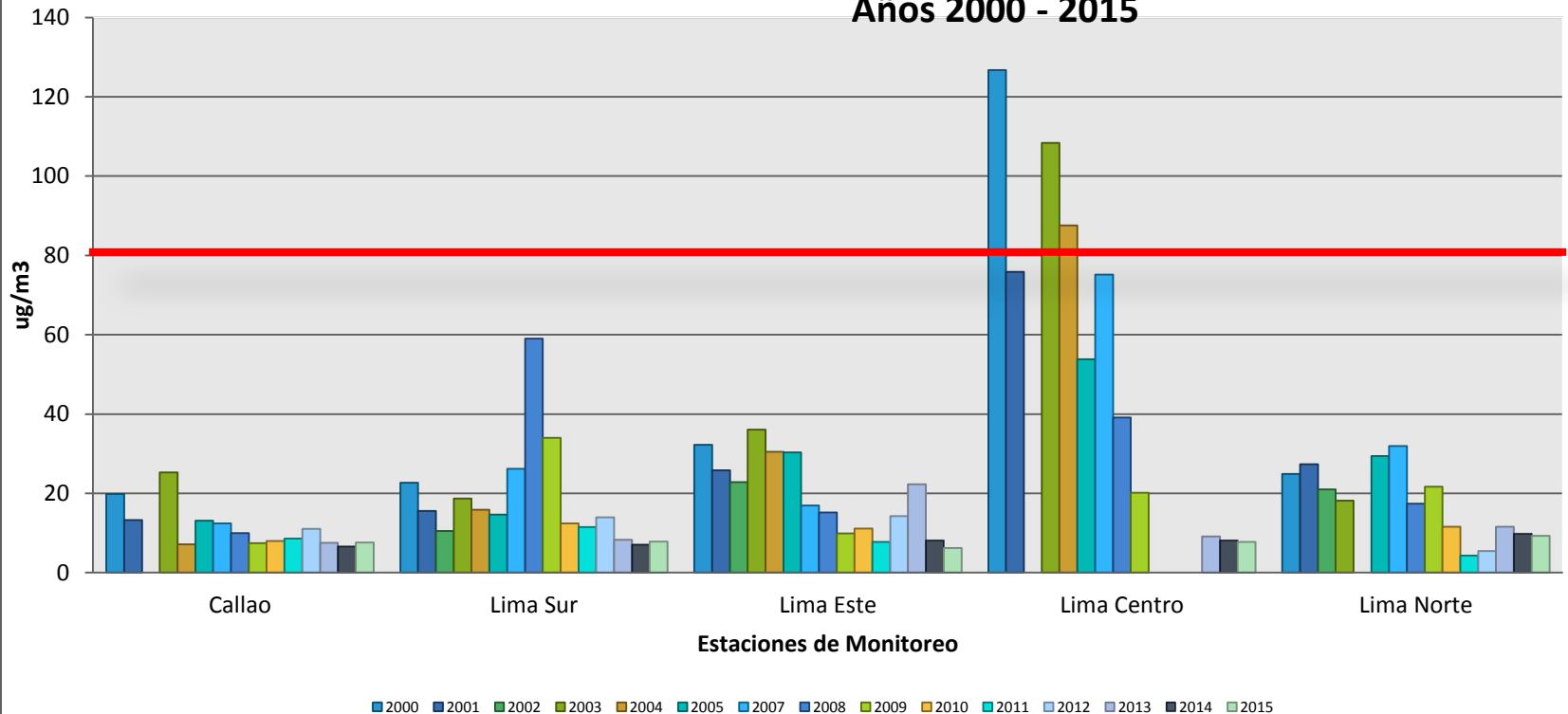
Comportamiento Anual del Dióxido de Azufre en las estaciones de la Red de Vigilancia en Lima -Callao Años 2000 - 2015
